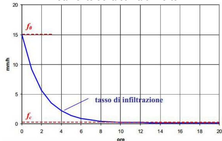
Andamento della curva di Horton
