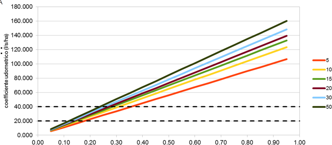
Coefficiente udometrico al variare del coefficiente di deflusso per ciascun tempo di ritorno (durata t=2 ore)
