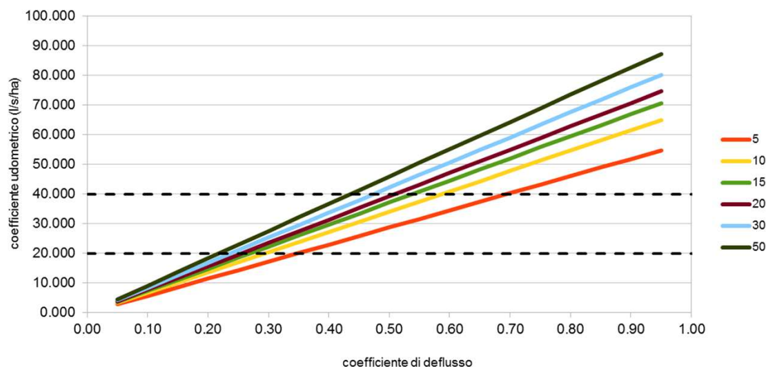
Coefficiente udometrico al variare del coefficiente di deflusso per ciascun tempo di ritorno (durata t=2 ore)
